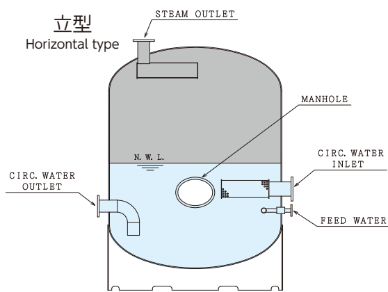
製品断面図 GENERAL VIEW
